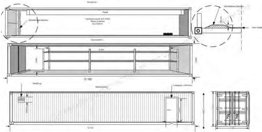
40' PSMC PFLANZENSCHUTZMITTEL LAGERCONTAINER DEPOT
